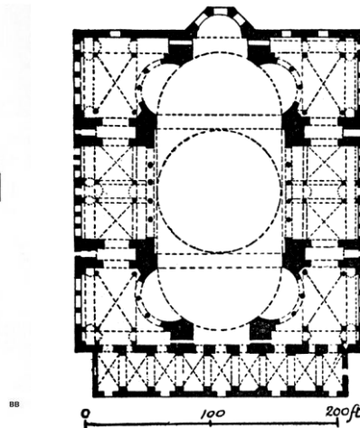
Grondplan Aya Sophia
